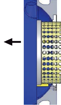
Ausführung mit Schlitz- oder Lochzylinder zum Regeln hoher Druckgefälle Exécution avec cylindre à fente ou perforé pour la régulation d'un gradient de pression élevé Esecuzione con cilindro a fessura o cilindro perforato per la regolazione di elevate cadute di pressione
