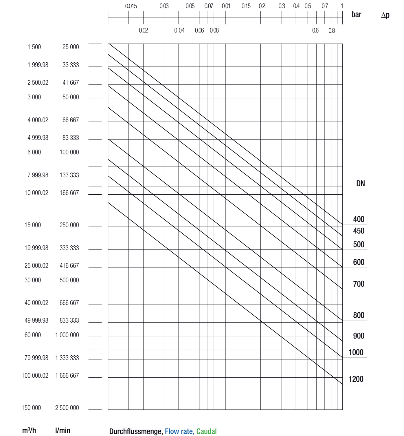
Druckverlustdiagramm DN 400 - 1200 unter Berücksichtigung Differenzdruck \Delta p Pressure loss diagram DN 400 - 1200 taking into account the differential pressure \Delta p Diagrama de pérdida de presión DN 400 - 1200 considerando la presión diferencial \Delta p
